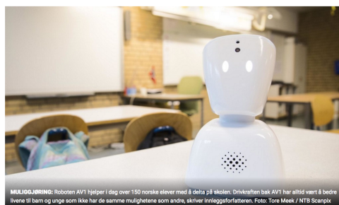
FILMER: Roboten AV1 skal gjøre det mulig for syke barn å være tilstede på skolen. Roboten streamer lyd og bilde fra klasserommet, og styres via en app. – Jeg finner det betenkelig at verden utenfor skal ha et kikkhull inn til der elever skal få prøve og feile, undannes og dannes, skriver innleggsgjortfateren. Foto: Tore Meek / NTB Scapix
