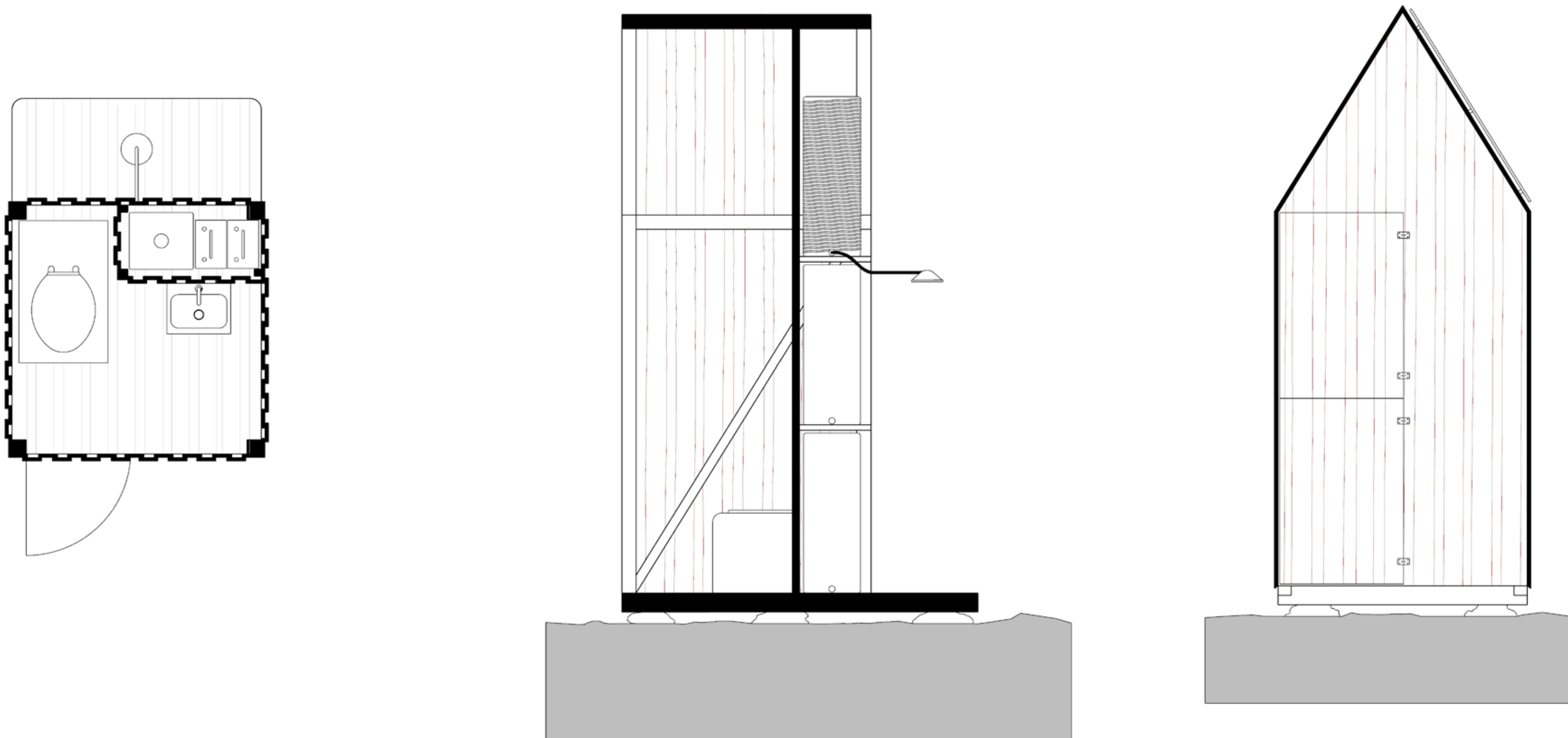
Plan 1:20
