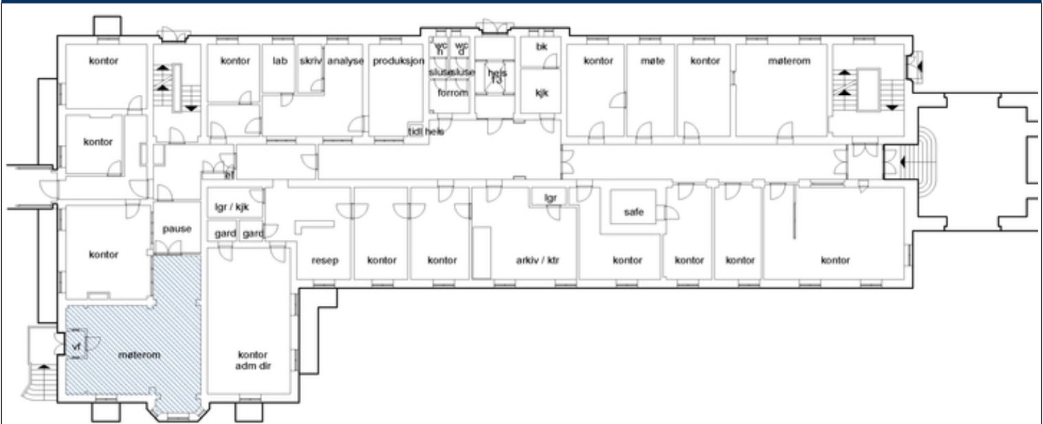
Plantegning 1. etasje, Administrasjonsbygningen. Omfang interiørfredning er markert med blå skravur.
